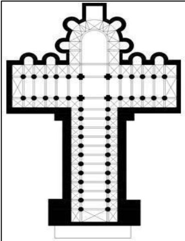
Planta de iglesia románica de peregrinación. Fuente: Wikimedia. Autor: Colomà. Licencia creative commons
