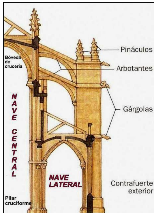
Sistema constructivo gótico. Autor: Carrillo Luque Fuente:Diccionarte. Licencia Creative Commons
